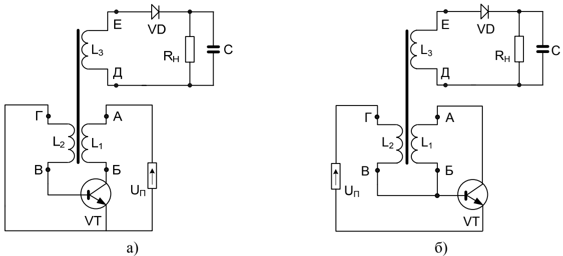
Рис. 6. Принципиальные электрические схемы качера-ТПТ.
