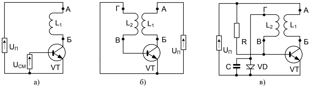
Рис. 3 Принципиальные электрические схемы качеров-УТ
