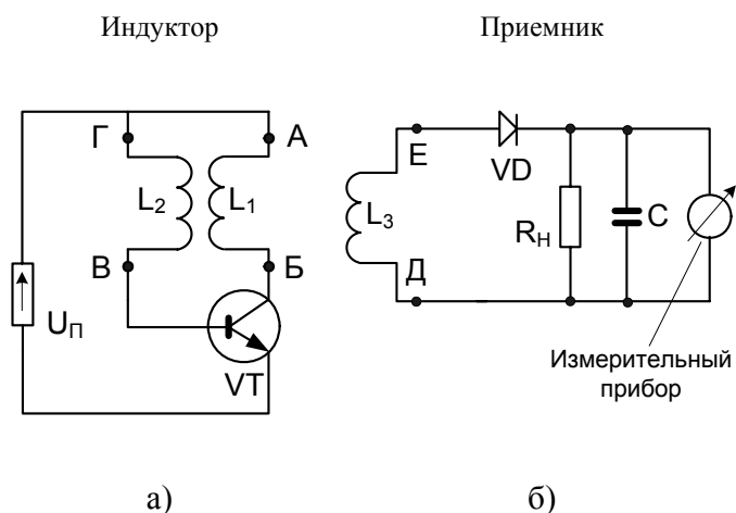
Рис. 2. Принципиальная электрическая схема одного из вариантов качера
