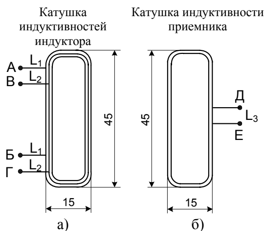
Рис. 1. Конструкция катушек индуктивностей качера
